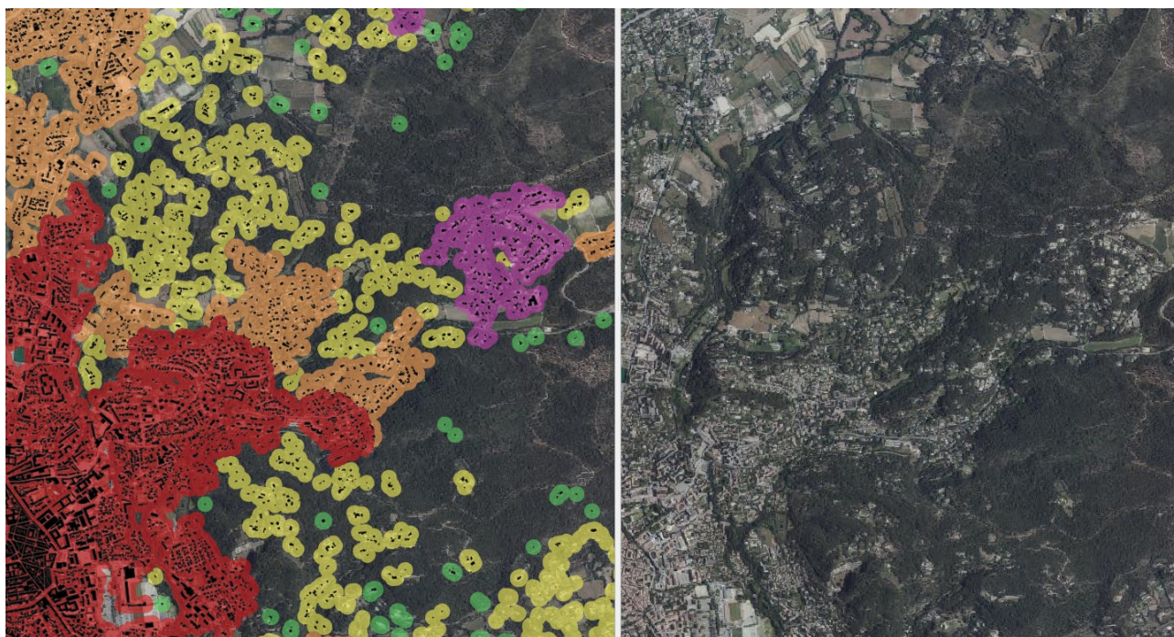
Illustration 16: Exemple de résultat de classification - méthode INRAE/ONF
