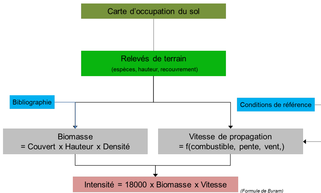
Illustration 15: Etapes de modélisation du combustible
